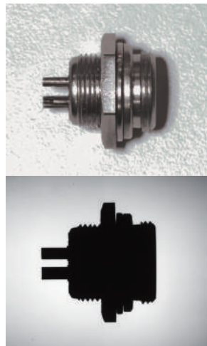
외형 및 치수 검사
