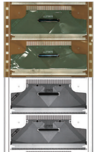
리드 프레임 및 패턴 검사
